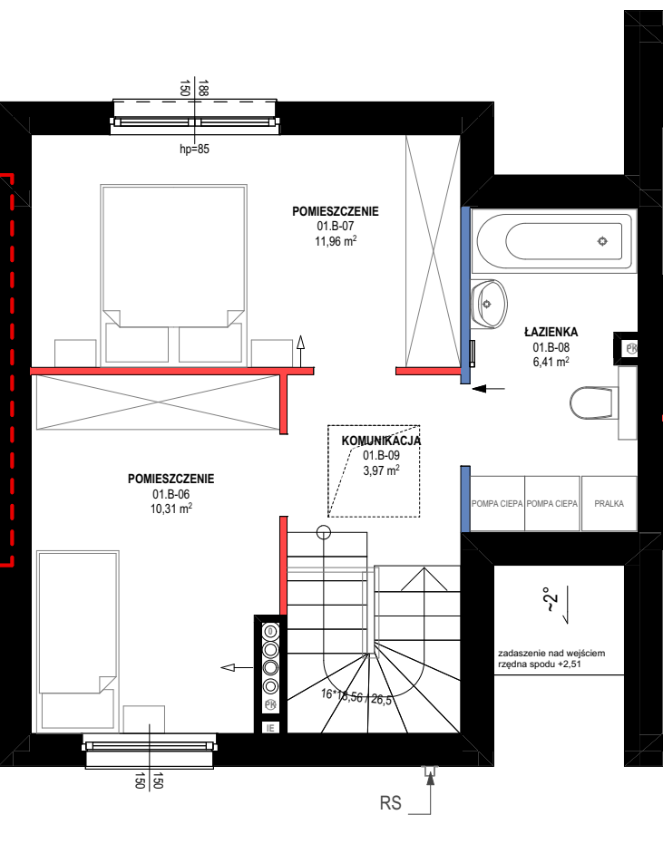
RZUT 1 PIĘTRA
