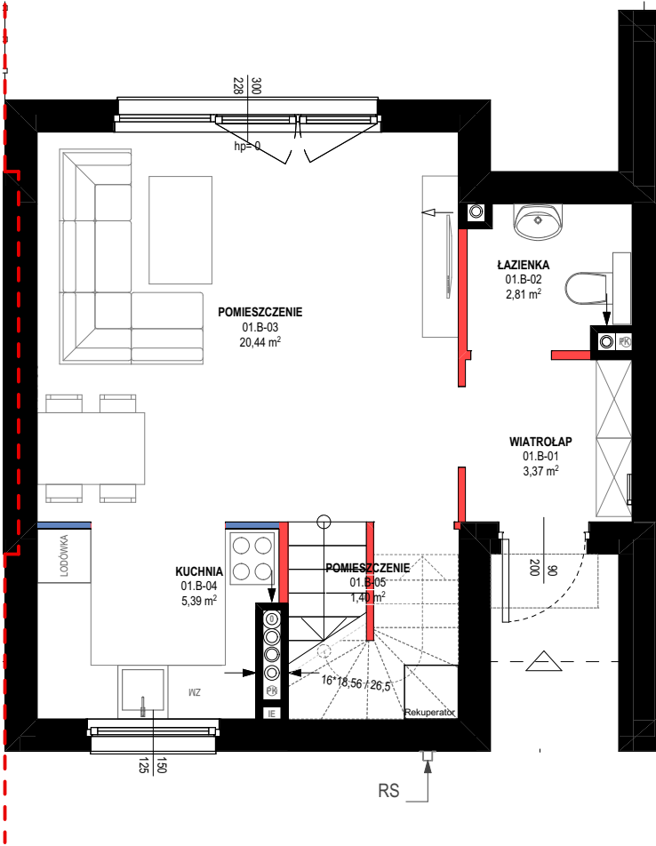
RZUT PARTERU
